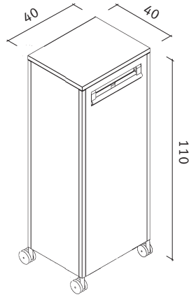
eQ Caddy
