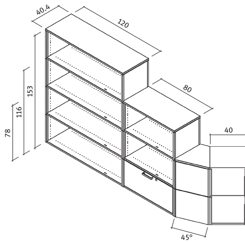
eQ Modul eQ Regalmodul 7/8 H
