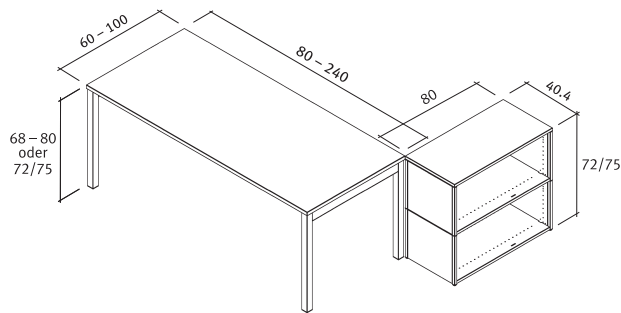
eQ Tisch eQ Tischmodul 7/8 H eQ Flex Table
